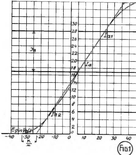
Fig. 1 = Kromme van de RE 504 bij 'n anodespanning van 150 Volt.
